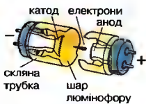
Газова лампа
